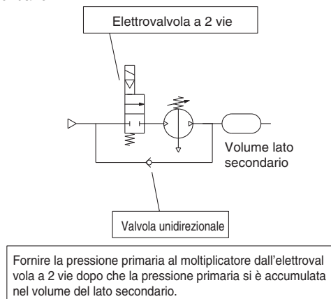
Circuito pneumatico raccomandato
