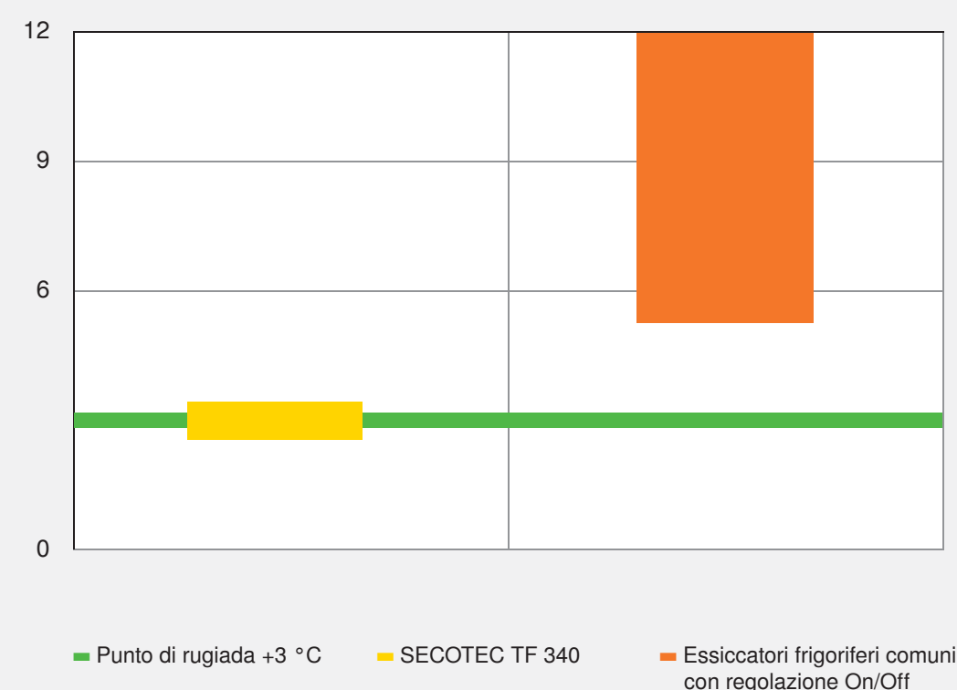
Grado di essiccazione espresso come punto di rugiada medio in °C
